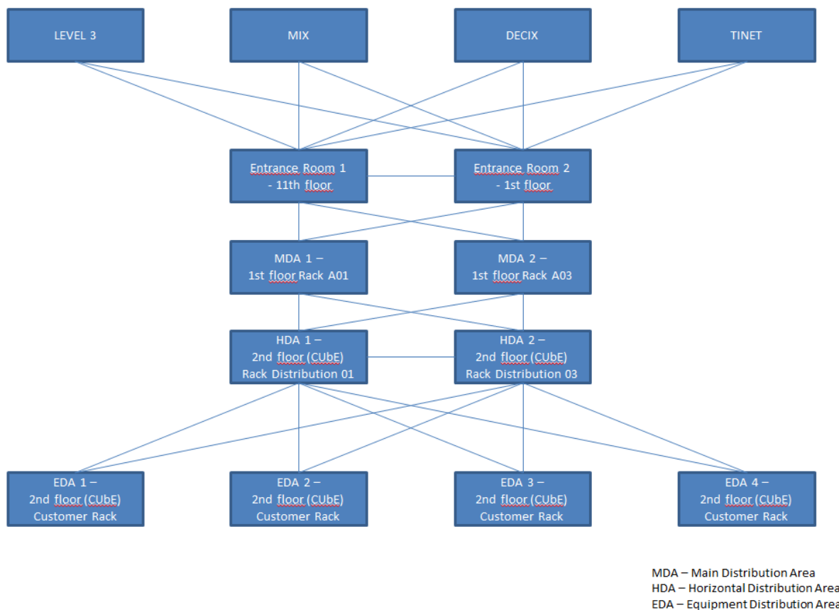
Figura 8 Struttura Data Center
